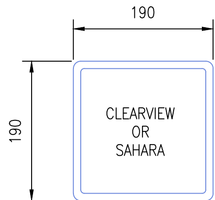
LENS PATTERN (SCALE=1:5.)
