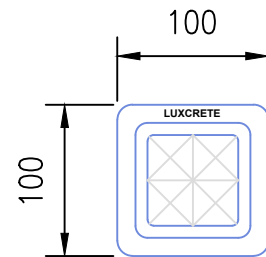
LENS PATTERN (SCALE=1:5.)
