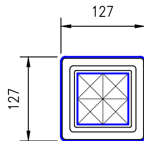
LENS PATTERN (SCALE=1:5.)
